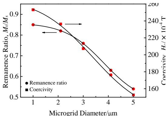
图 5 剩磁比及矫顽力与孔径之间的关系
