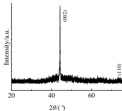
图 3 原 56.7 nm Co 薄膜的 XRD 图谱
