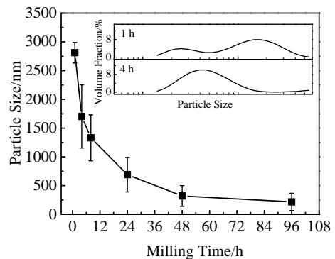
图 2 颗粒尺寸随球磨时间的变化
