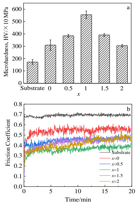
图 8 FeCo x CrAlCu 高熵合金涂层和 45#钢基体的显微硬度和摩擦系数
