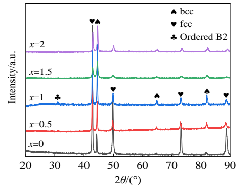
图 4 FeCo x CrAlCu 高熵合金涂层的 XRD 图谱 Fig.4 XRD patterns of FeCo x CrAlCu high entropy alloy coating
