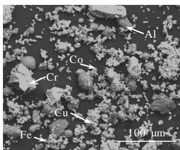
图 1 冷喷涂预制粉末微观形貌
