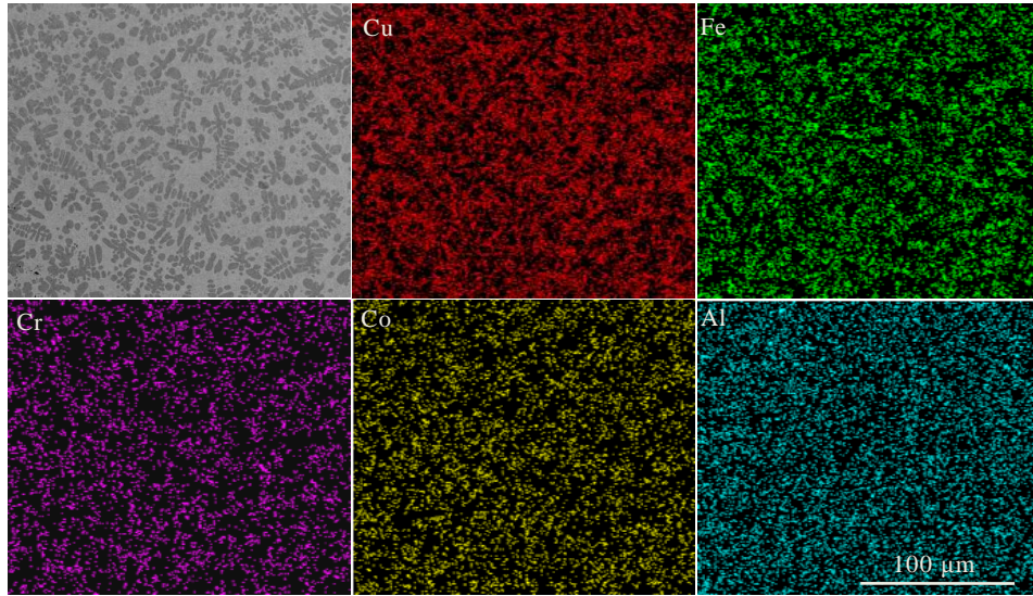
图 7 FeCo 0.5 CrAlCu 高熵合金涂层形貌及 EDS 元素面扫描
