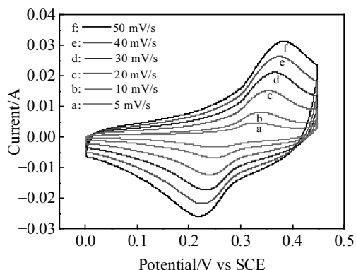
图 5 碳包覆氧化镍纳米颗粒在不同扫描速度下的循环伏安曲线
