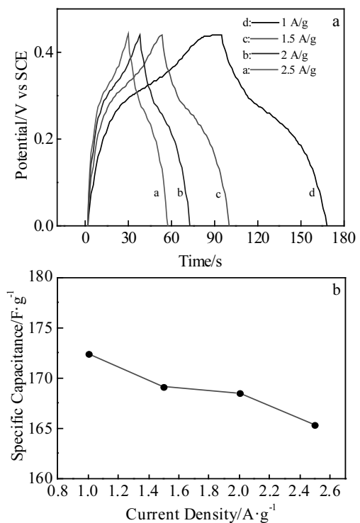
图 6 碳包覆氧化镍纳米颗粒在不同电流密度下的充放电曲线和比电容值
