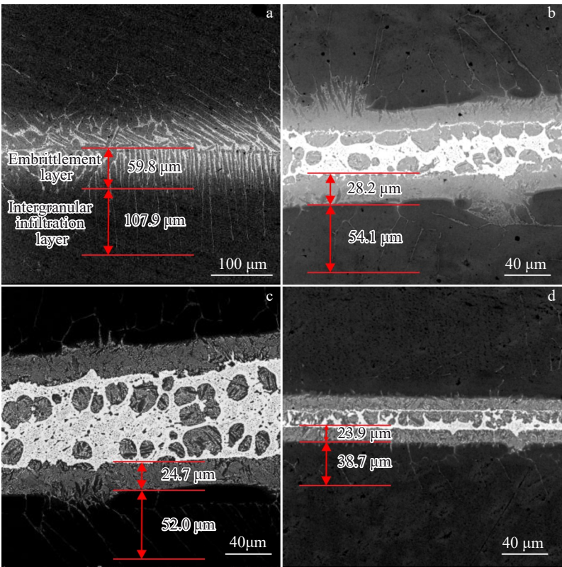
图 2 TA2 钛合金钎焊接头界面元素扩散距离(保温时间 15 min)
