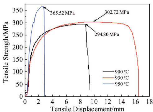
图4 TA2钛合金钎焊接头抗拉强度与钎焊温度的关系
