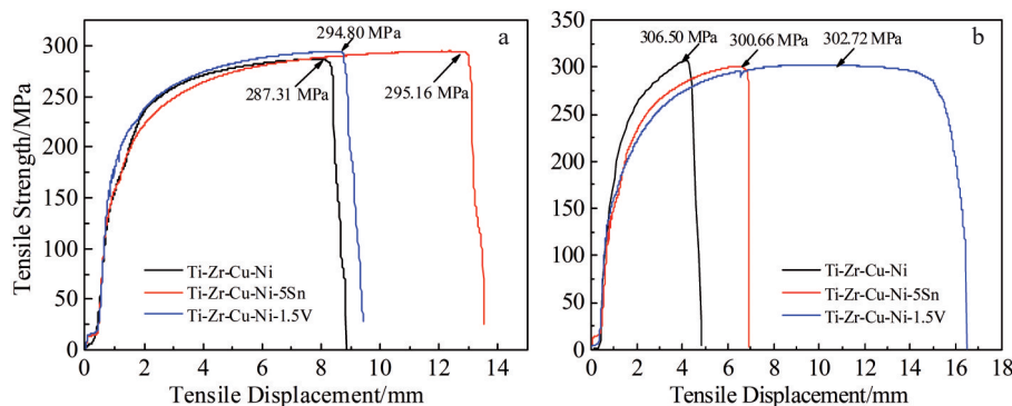
图3 TA2钛合金钎焊接头抗拉强度与钎料成分的关系
