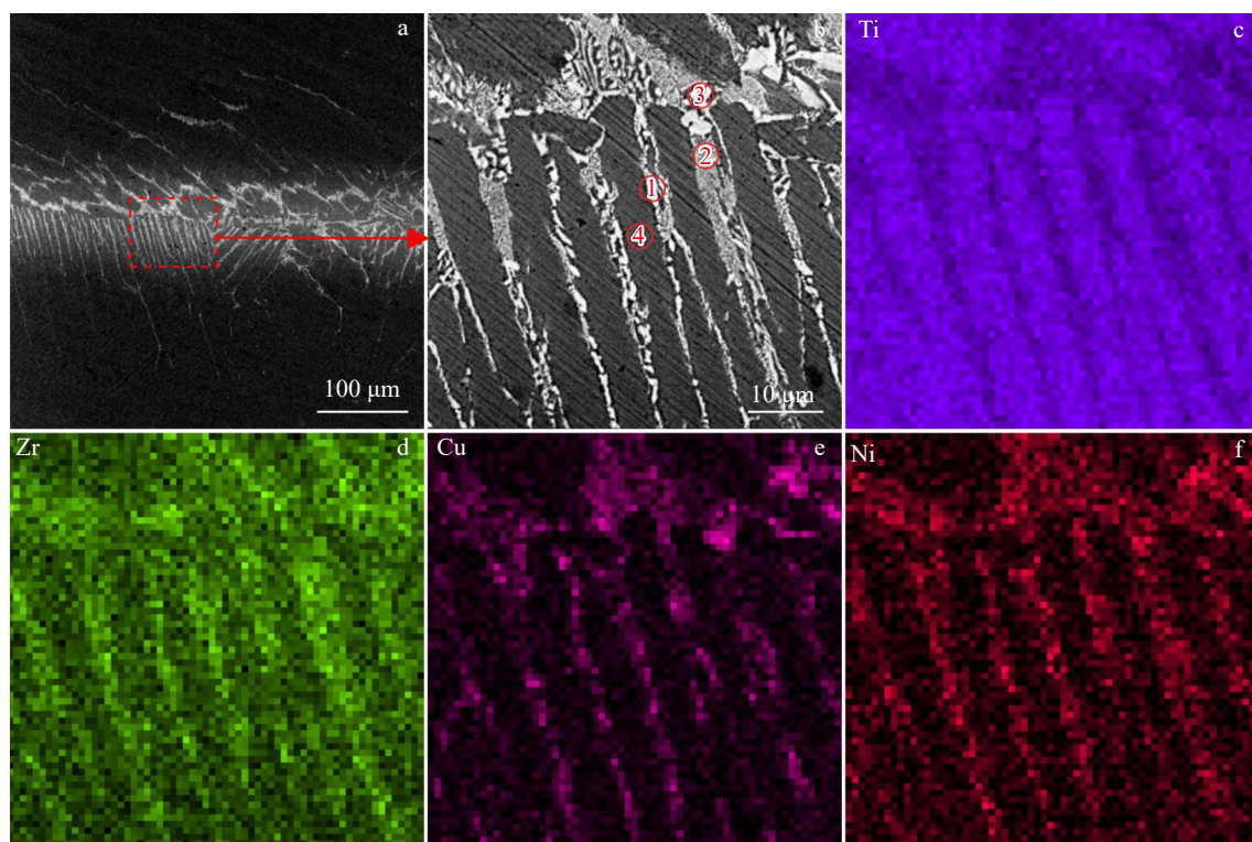
图1 TA2钛合金钎焊接头SEM照片及EDS元素面扫描
