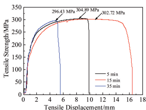
图5 TA2钛合金钎焊接头抗拉强度与保温时间的关系
