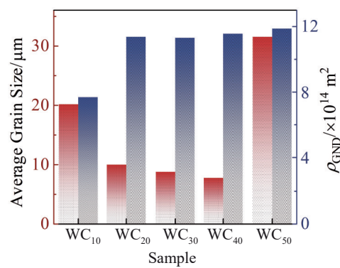
图7 晶粒平均尺寸和几何必须位错密度 Fig.7 Average grain size and the value of \rho_{\text{GND}}
