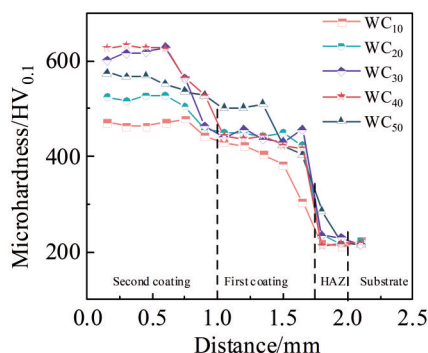
图8 涂层沿深度方向的显微硬度分布
