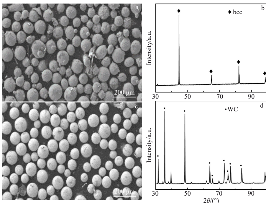
图1 AlCoCrFeNi 合金粉末的形貌和 X 射线衍射图谱; 球形 WC 粉的形貌和 X 射线衍射图谱
