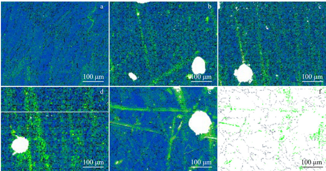
图6 涂层局部取向差图
