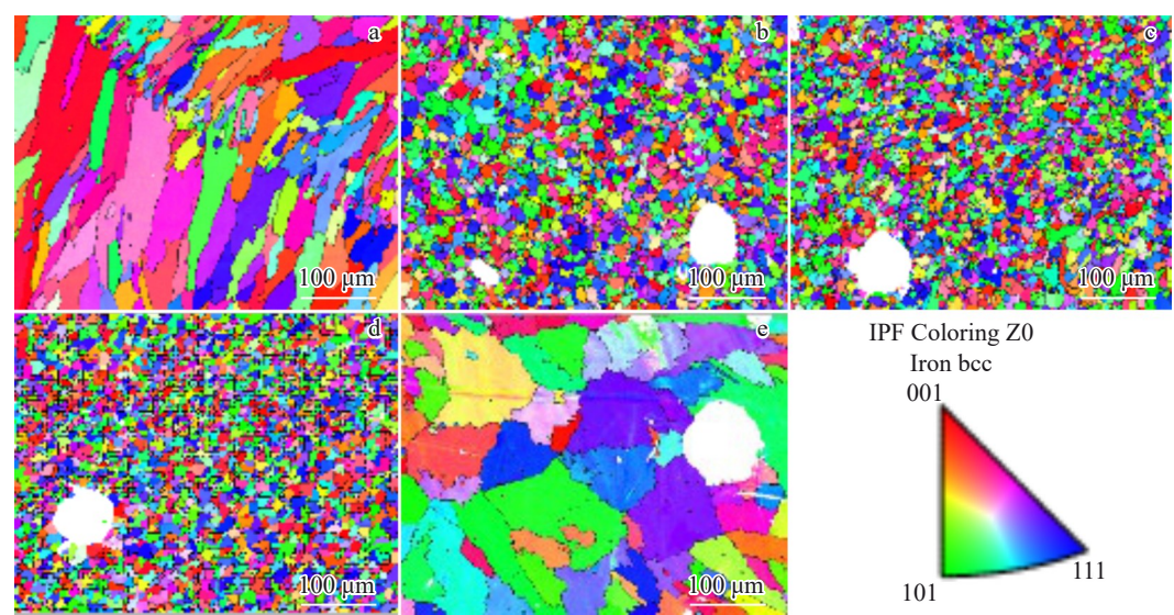
图5 涂层反极图
