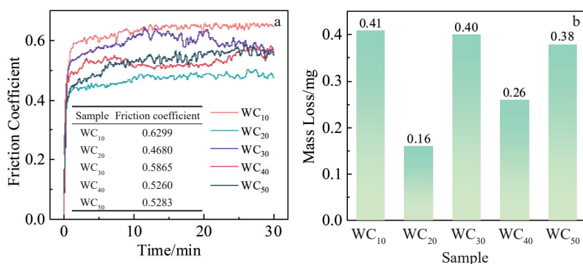
图9 各涂层摩擦系数曲线以及样品在摩擦测试过程中的质量损失
