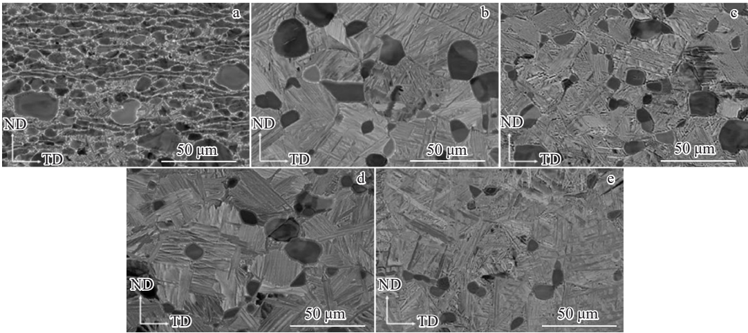
图7 换向轧 \delta 1 mm板材不同热处理条件下的微观组织形貌
