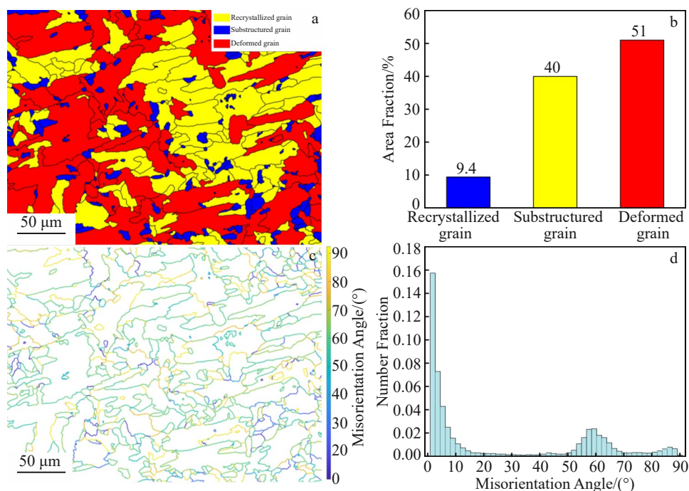
图 3 \delta 32\ \text{mm} 板材再结晶特征及界面取向差分析
