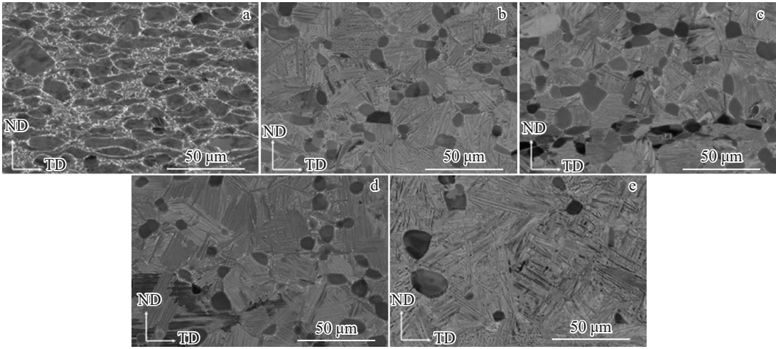
图8 顺轧 \delta 1 mm板材不同热处理条件下的微观组织形貌
