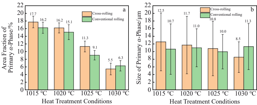
图9 不同温度固溶后时效700 °C/4 h 初生 \alpha 相统计结果
