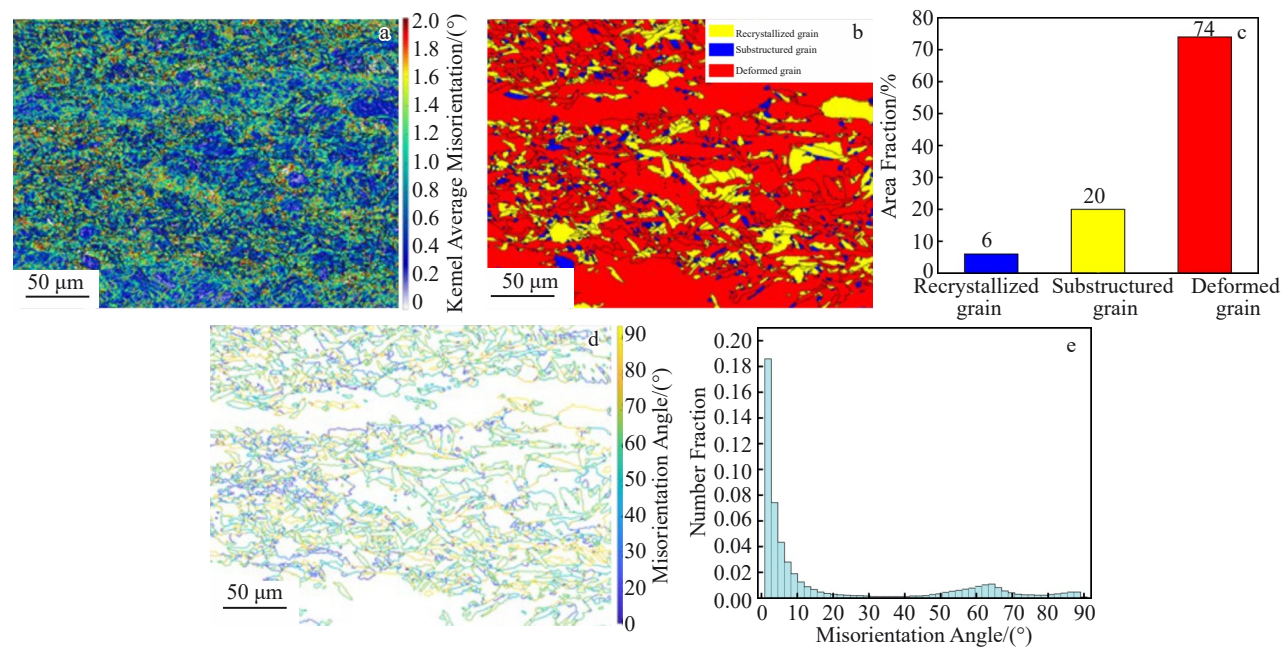
图5 δ10 mm 板材再结晶特征及界面取向差分析
