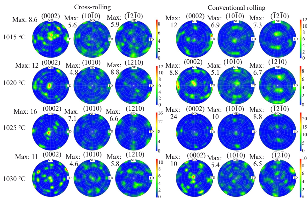
图 11 不同固溶温度热处理后 \delta 1 mm 板材极图
