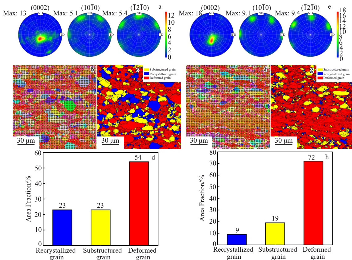
图6 \delta 1 mm 板材组织表征结果
