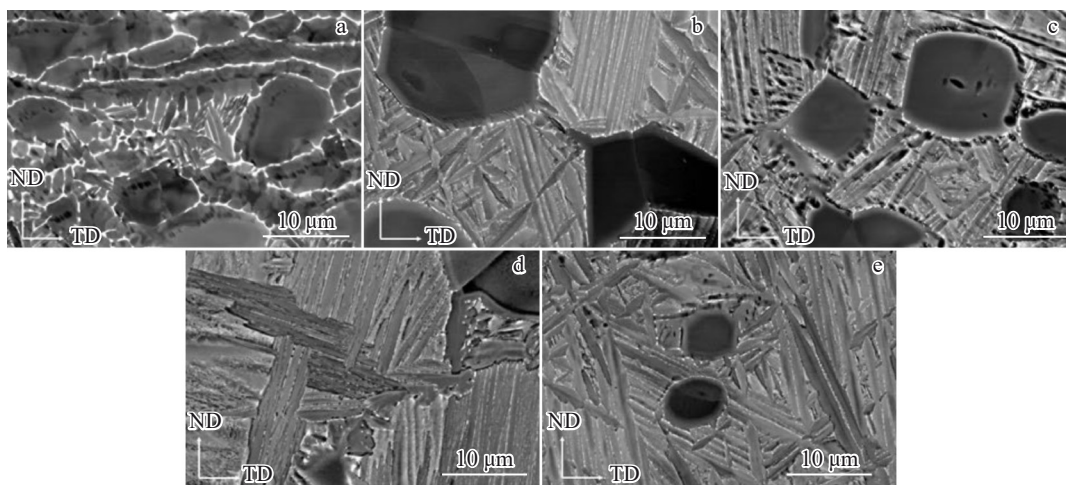
图 10 换向轧 \delta 1 mm 板材不同热处理条件下的析出行为
