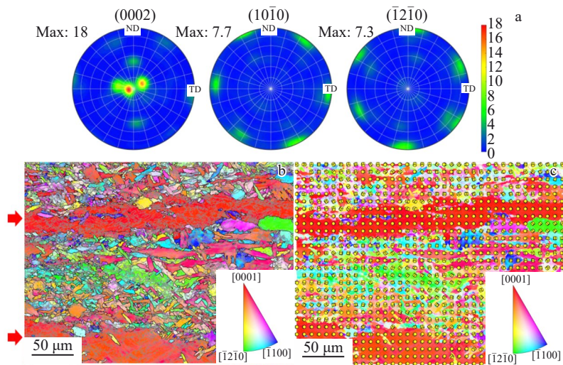
图4 δ10 mm 板材织构表征结果
