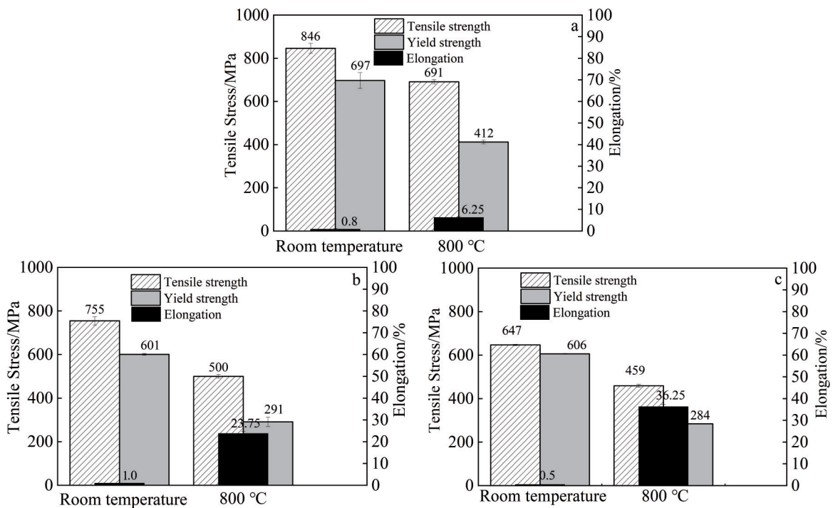
图7 TMMW合金的拉伸性能
