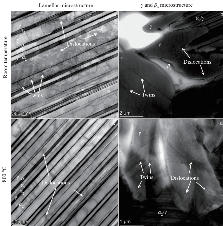
图 13 拉伸试验后 HT1 变形组织中位错分布的 TEM 明场像
