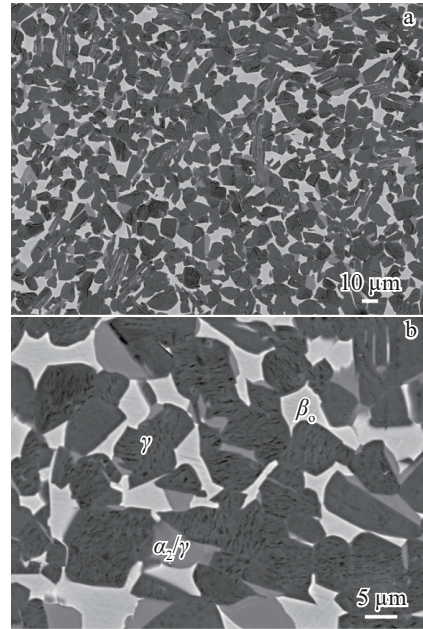
图3 TMMW 合金的初始组织
