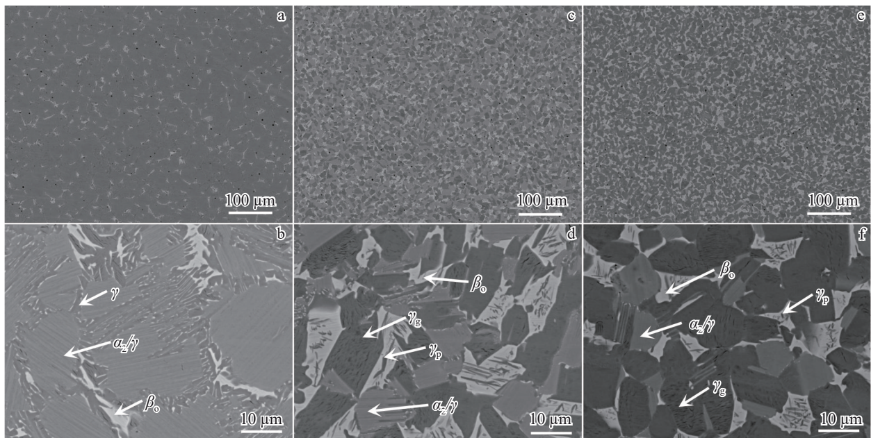
图4 TMMW 合金的EPMA 照片
