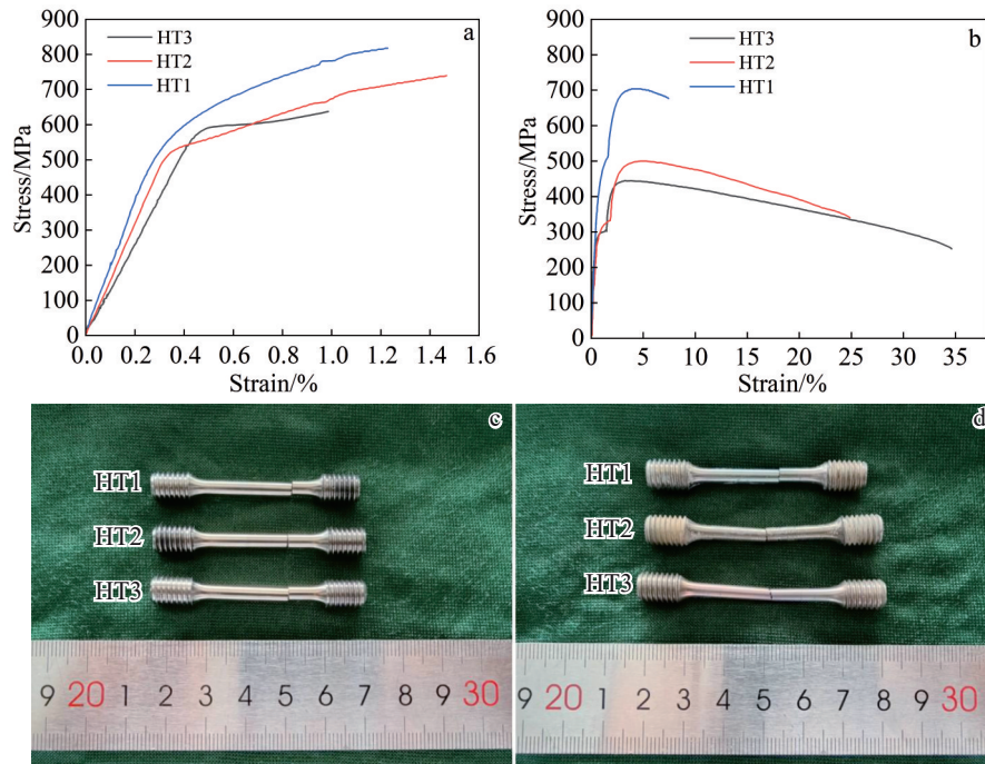
图8 TMMW 合金的拉伸应力-应变曲线和拉伸试样外观(实物图)
