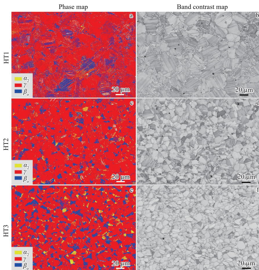
图6 TMMW合金的EBSD照片
