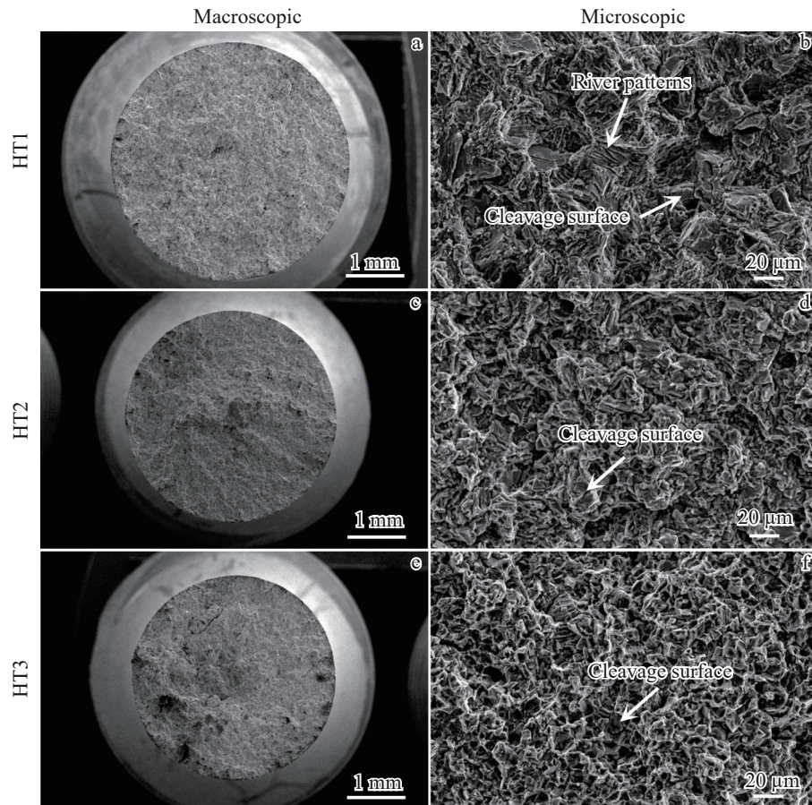
图10 TMMW合金800℃宏观及微观拉伸断口形貌
