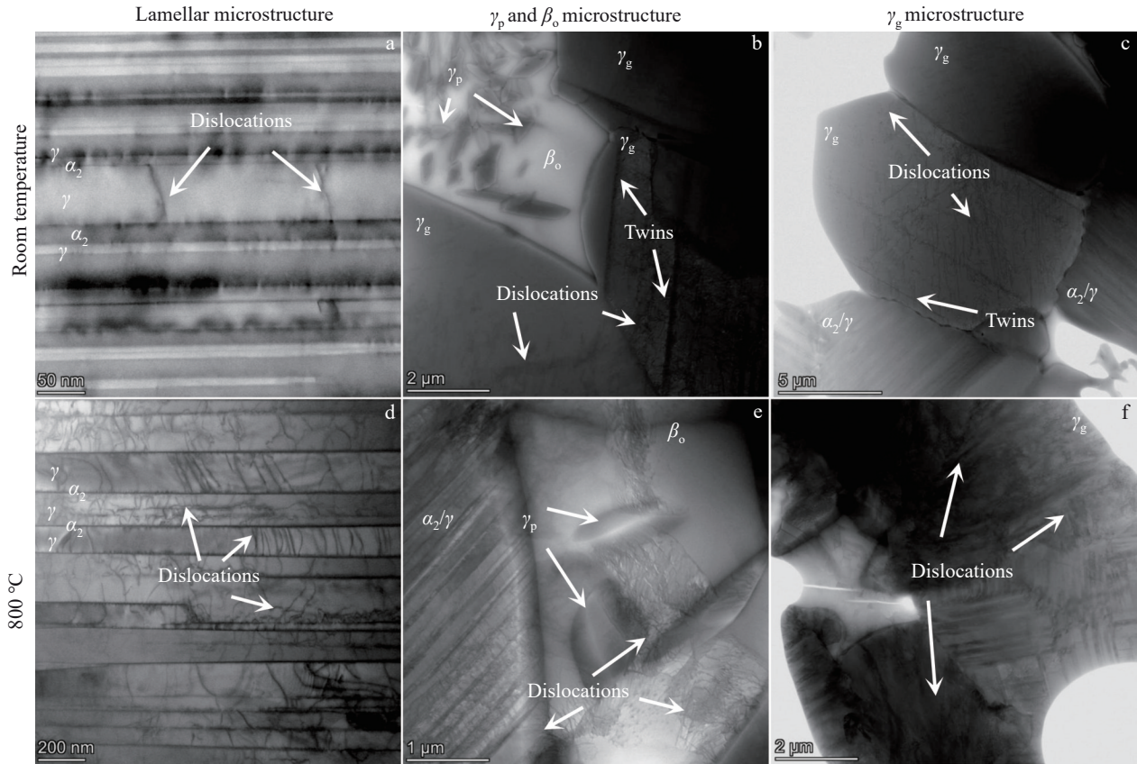
图 14 拉伸试验后 HT3 变形组织中位错分布的 TEM 明场像
