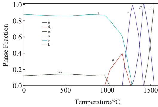
图2 TMMW 合金的平衡相图
