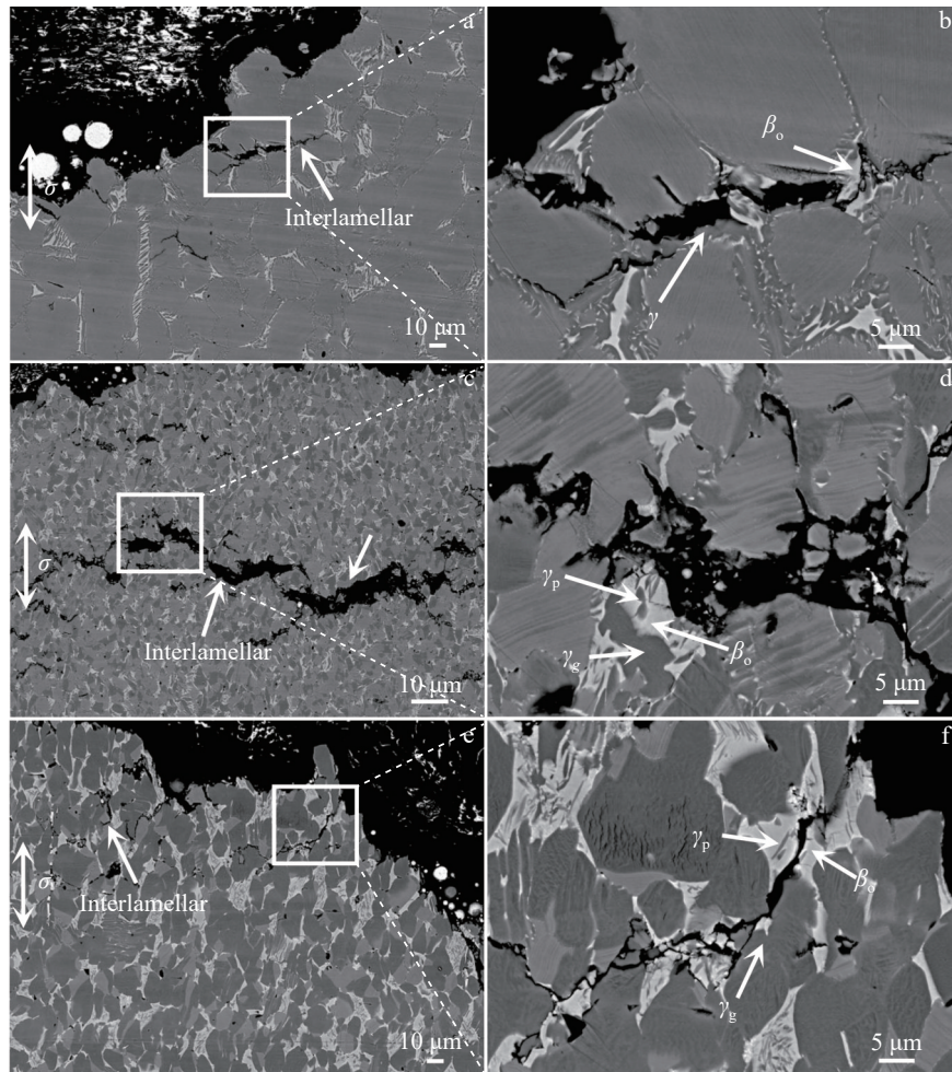
图12 TMMW合金800 °C拉伸断口纵剖面的显微组织
