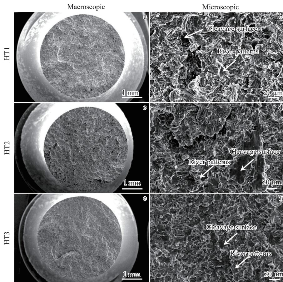
图9 TMMW 合金室温宏观及微观拉伸断口形貌
