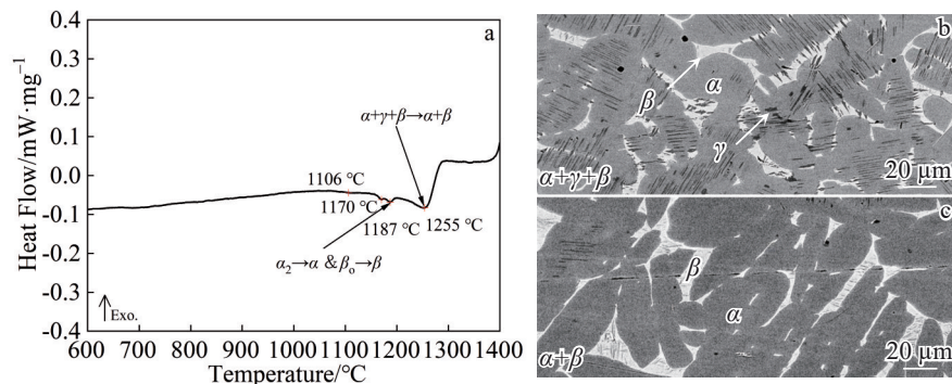
图1 TMMW合金的DSC曲线和水淬组织的EPMA照片
