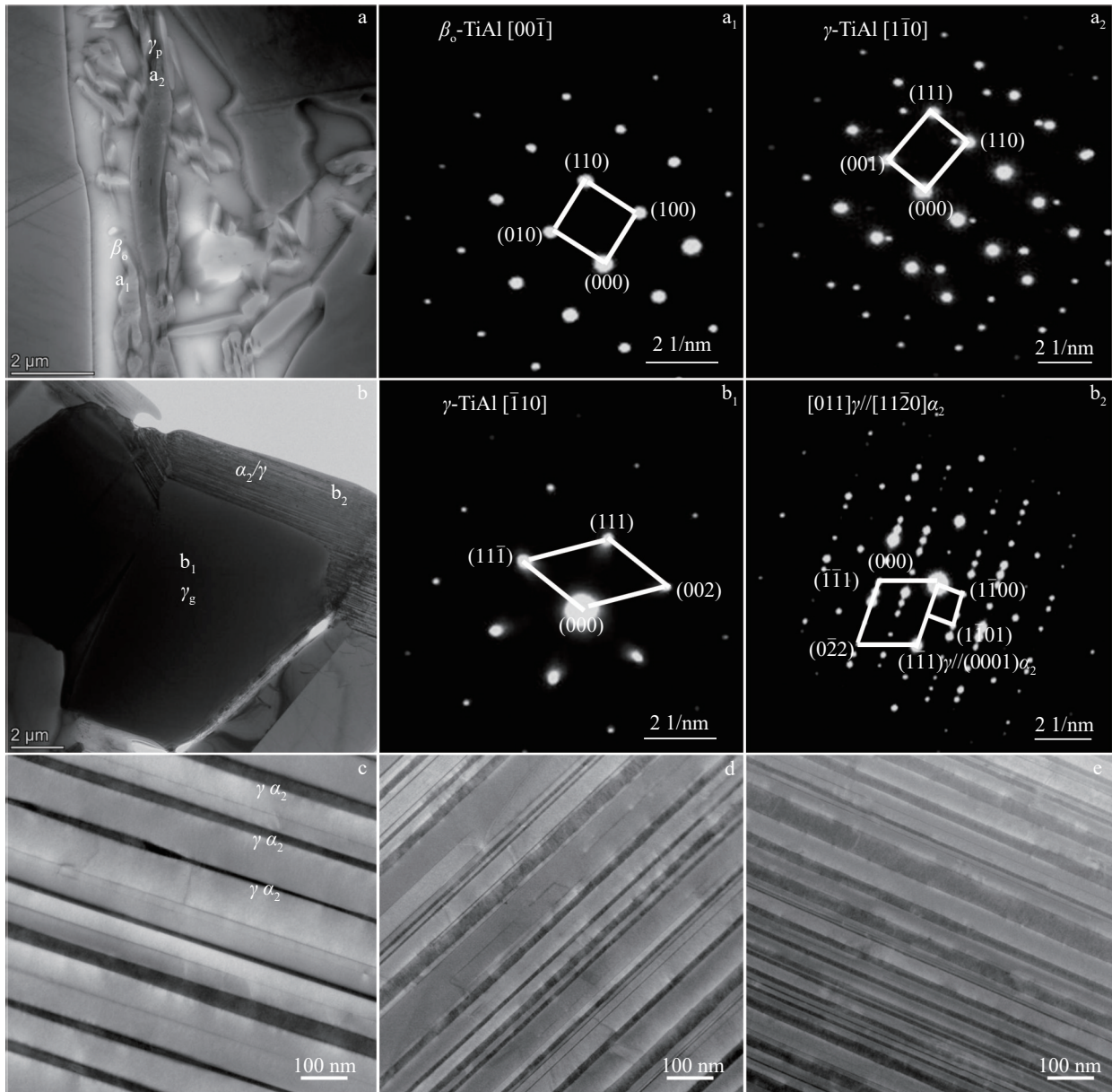
图5 TMMW合金的TEM分析
