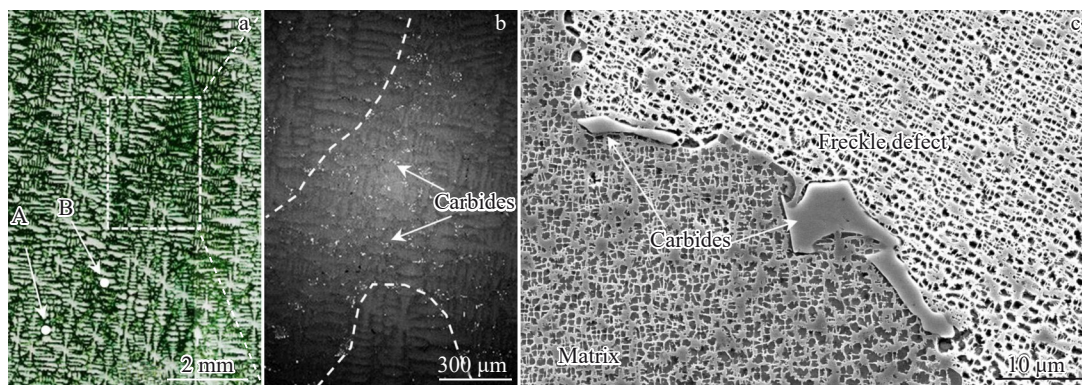
图5 保温温度 1490 °C 下某雀斑缺陷前沿沟槽偏析微观形貌
