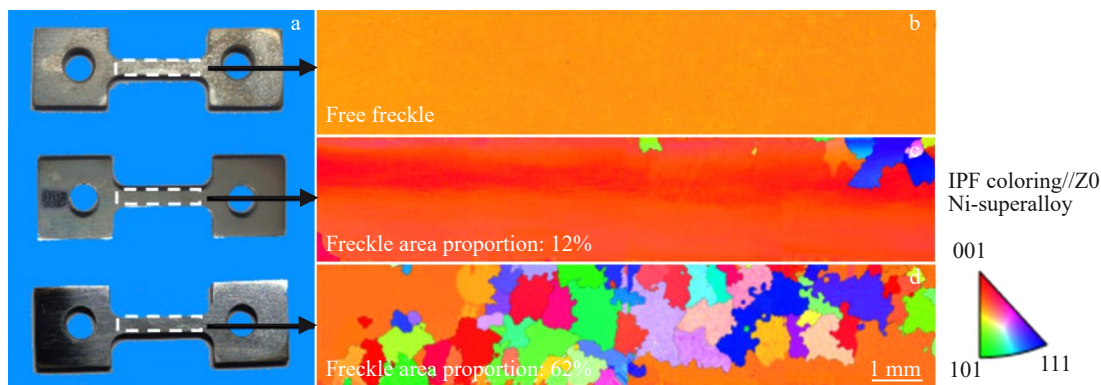
图 12 不同高温持久实验的试样标距段的取向面分布图
