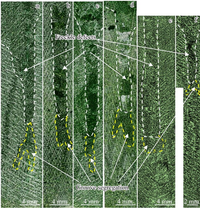
图4 不同保温温度下 S1 区域(图 2)某雀斑缺陷放大图
