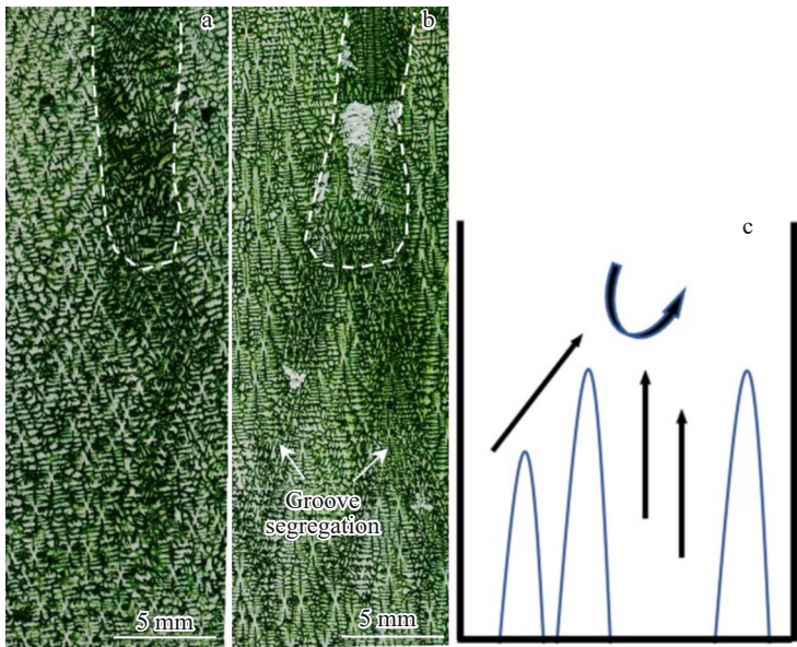
图 11 熔液密度反转导致的熔液对流和通道合并导致的熔液对流形貌及通道合并导致的熔液对流示意图
