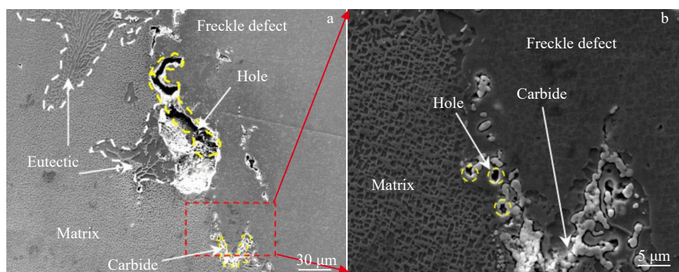
图 13 热处理后晶界处残余共晶和共晶区域放大图
