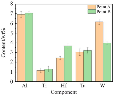
图7 图5a中不同点位处残余液相成分含量
