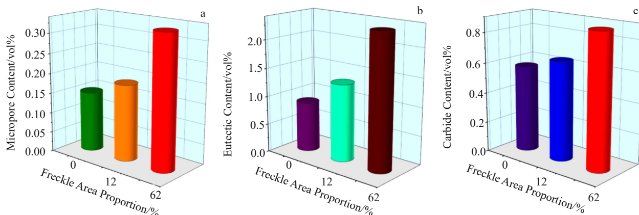
图 17 不同雀斑面积占比试样的微孔体积分数、共晶含量和碳化物含量
