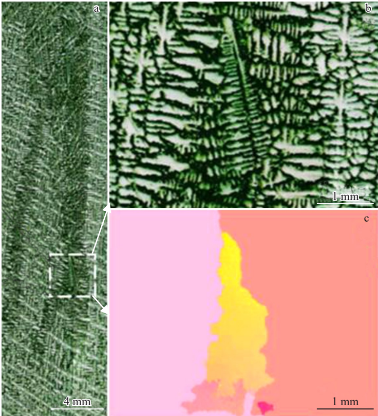
图 10 雀斑缺陷放大图、沟槽偏析内断裂枝晶和断裂枝晶 EBSD 图
