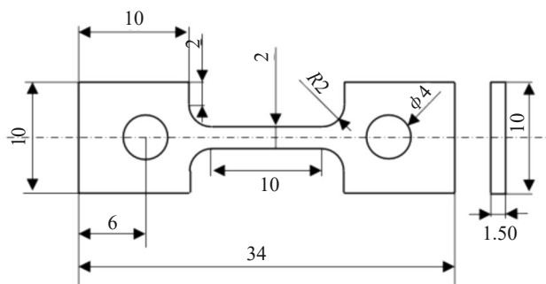
图1 板状持久试样尺寸示意图
