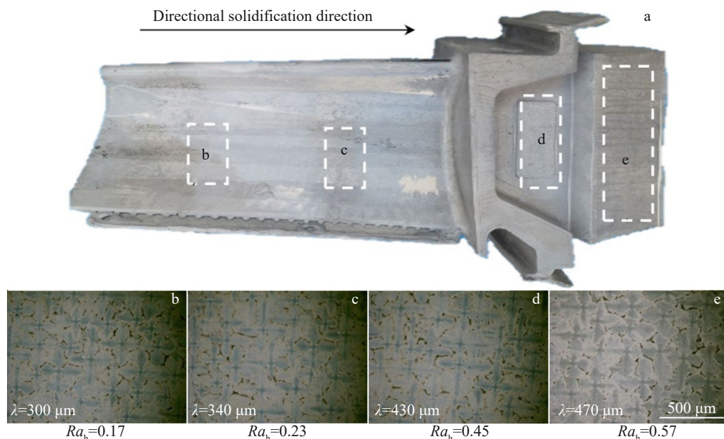
图9 不同叶片高度横截面微观组织及瑞利数
