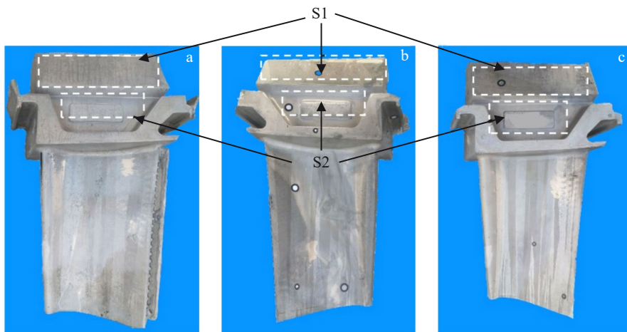
图2 不同保温温度下大尺寸叶片宏观形貌图
