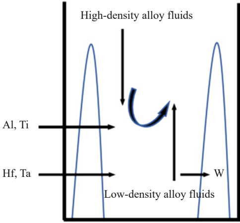
图8 熔液密度反转导致的熔液对流机理示意图
