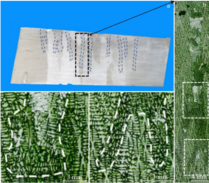
图3 保温温度 1500 ℃下 S1 区域(图 2b)某雀斑缺陷宏观形貌
