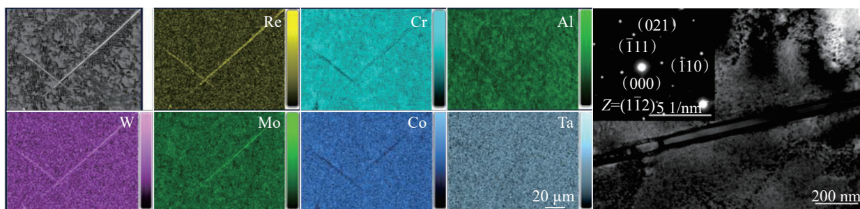
图 12 TCP 相的 SEM 照片, EDS 元素面扫描和 TEM 衍射斑点的标定
