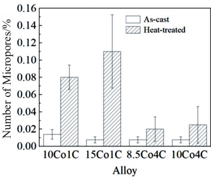
图2 热处理前后 4 种合金的微孔数量
