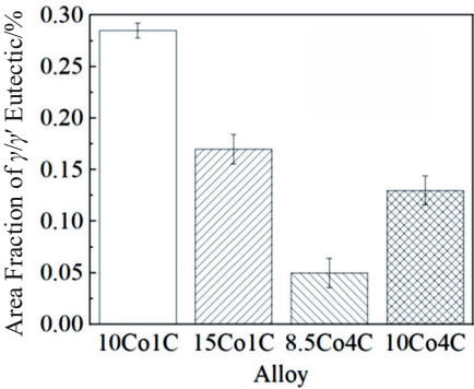
图4 4 种合金铸态组织中的共晶含量 Fig.4 Eutectic content in microstructure of four as-cast alloys
