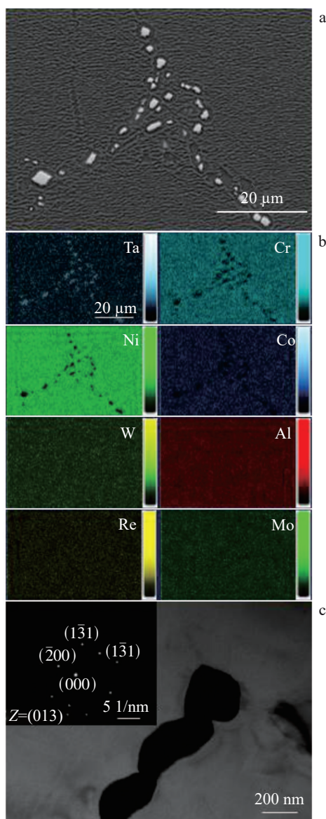
图5 MC型碳化物的SEM照片和EDS元素面扫描及TEM衍射斑点标定
