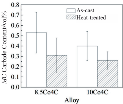
图3 热处理前后 8.5Co4C 合金和 10Co4C 合金的 MC 碳化物含量 Fig.3 Content of MC carbides in 8.5Co4C alloy and 10Co4C alloy before and after heat treatment
