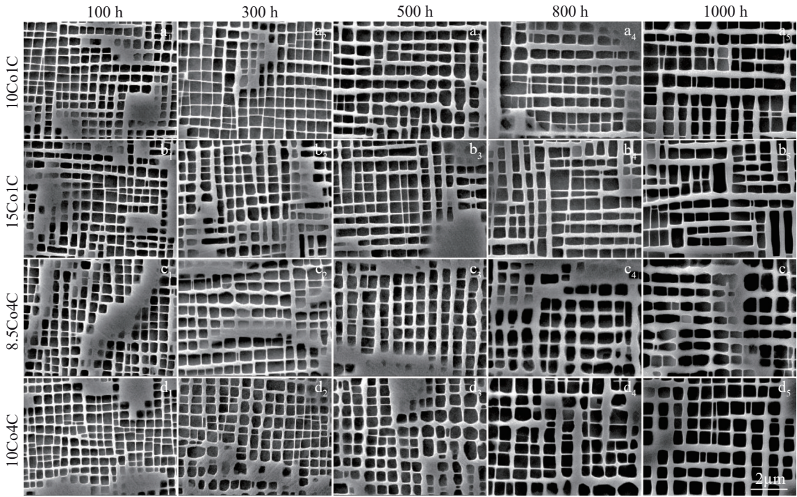
图9 4种合金 \gamma' 相形貌随时效时间的变化
