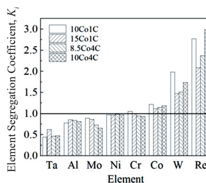
图6 4种合金铸态下各元素的偏析系数
