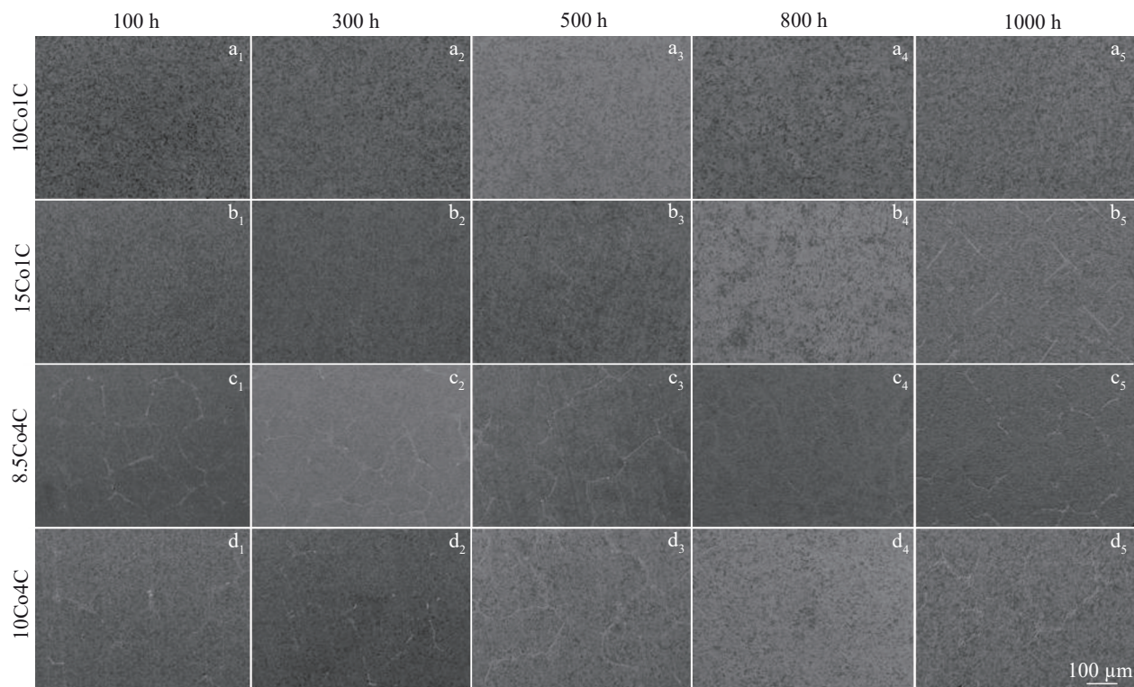
图 11 4 种合金在 1000 °C 长期时效过程中 TCP 相的析出形貌
