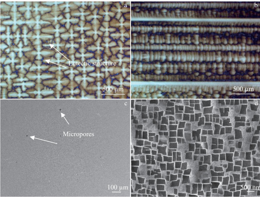
图1 8.5Co4C 合金的铸态组织形貌
