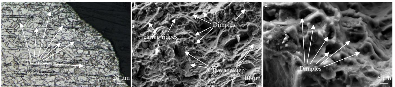
图 7 挤压态 AZXVM80100 合金断口组织与断口形貌: (a) 挤压态 AZXVM80100 合金拉伸断口 OM 组织; (b, c) 挤压态
