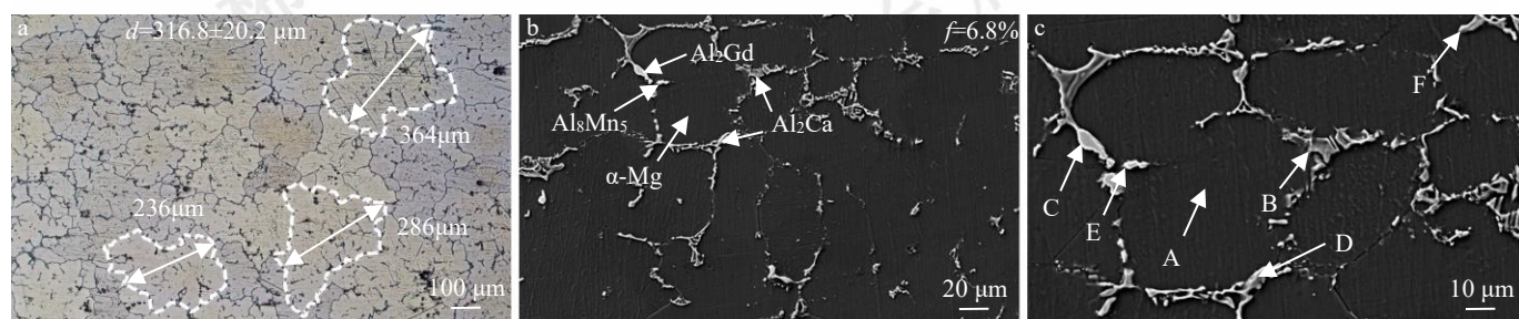
图 1 固溶态 AZXVM80100 合金微观组织: (a) OM; (b, c) SEM
