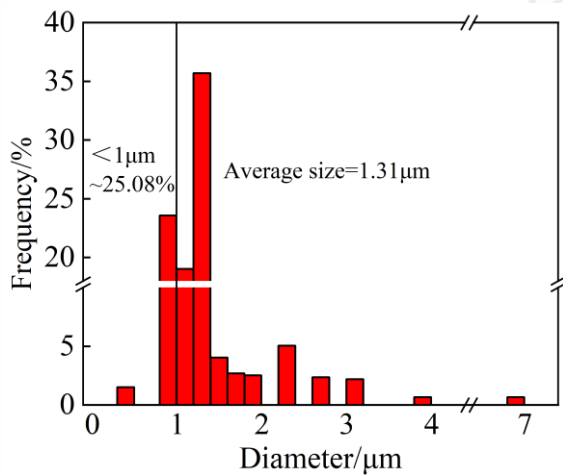
图4 挤压态 AZXVM80100 合金中第二相尺寸分布图
