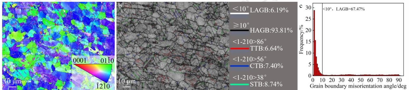
图 8 拉伸应变为 8%时挤压态 AZXVM80100 合金的 EBSD 组织: (a) 8%应变 AZXVM80100 合金 IPF 组织; (b) 8%应变 AZXVM80100 合金 GB 图与不同类型晶界比例; (c) 不同取向差晶界比例分布图
