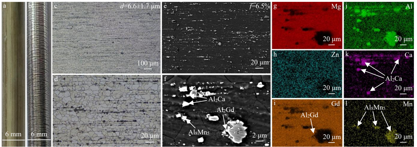
图3 高速 (32.4) m/min 挤压 AZXVM80100 合金的表面宏观形貌与微观组织特征: (a) 高速挤压 AZXVM80100 合金宏观照片; (b) 高速挤压 AZ80 合金宏观照片; (c, d) 挤压态 AZXVM80100 合金 OM 组织; (e, f) 挤压态 AZXVM80100 合金 SEM 组织; (g-l) 挤压态 AZXVM80100 合金 EDS 面分析结果
