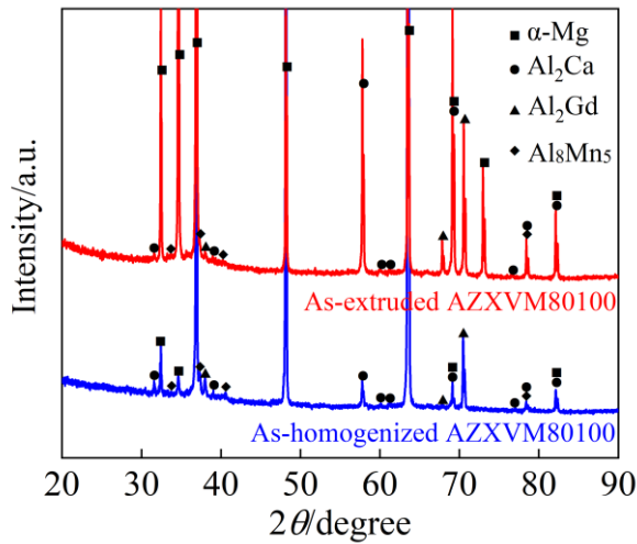
图 2 固溶态与挤压态 AZXVM80100 合金的 XRD 谱
