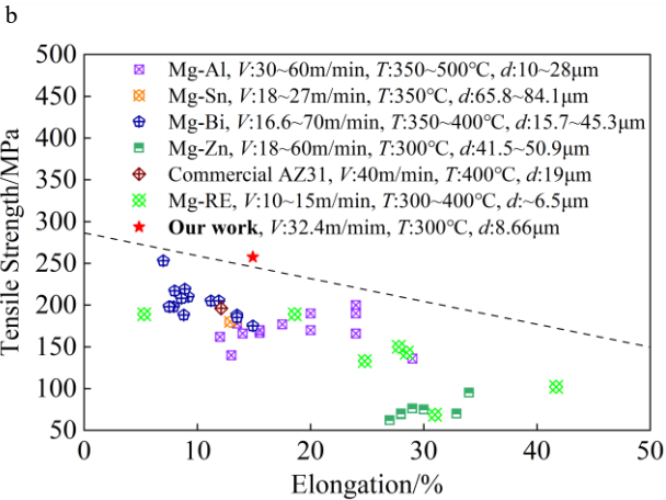
图 6 AZXVM80100 合金的力学性能及其与其它高速挤压镁合金强塑性能对比 [15,18-25,31-42] ：(a) 挤压态与固溶态 AZXVM80100 合金典型拉伸工程应力-应变曲线；(b) 高速(10~70 m/min)挤压镁合金屈服强度与延伸率对比图 [15,18-25,31-42]
