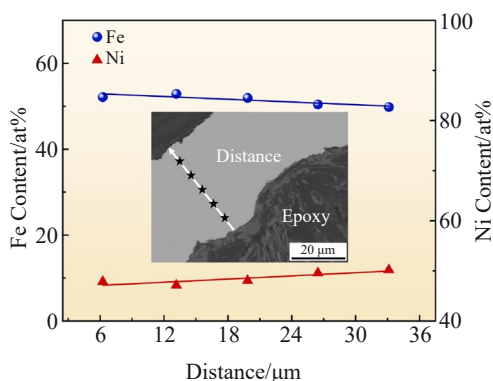
图8 多孔Ni-Fe合金的元素分布
