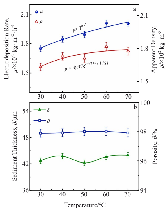
图4 不同沉积温度下多孔 Ni-Fe 合金的结构参数
