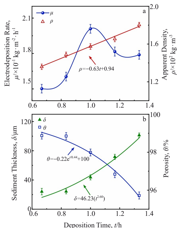
图5 多孔 Ni-Fe 合金的沉积速率、表观密度、沉积层厚度及孔隙率随沉积时间的变化曲线
