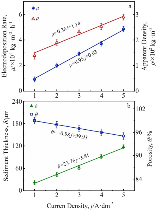
图3 阴极电流密度对多孔 Ni-Fe 合金结构特征的影响
