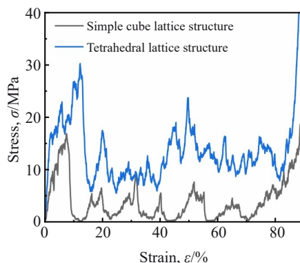
图9 多孔Ni-Fe合金的应力-应变曲线
