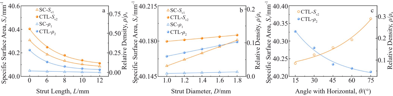
图2 杆元参数对点阵结构比表面积和相对密度的影响
