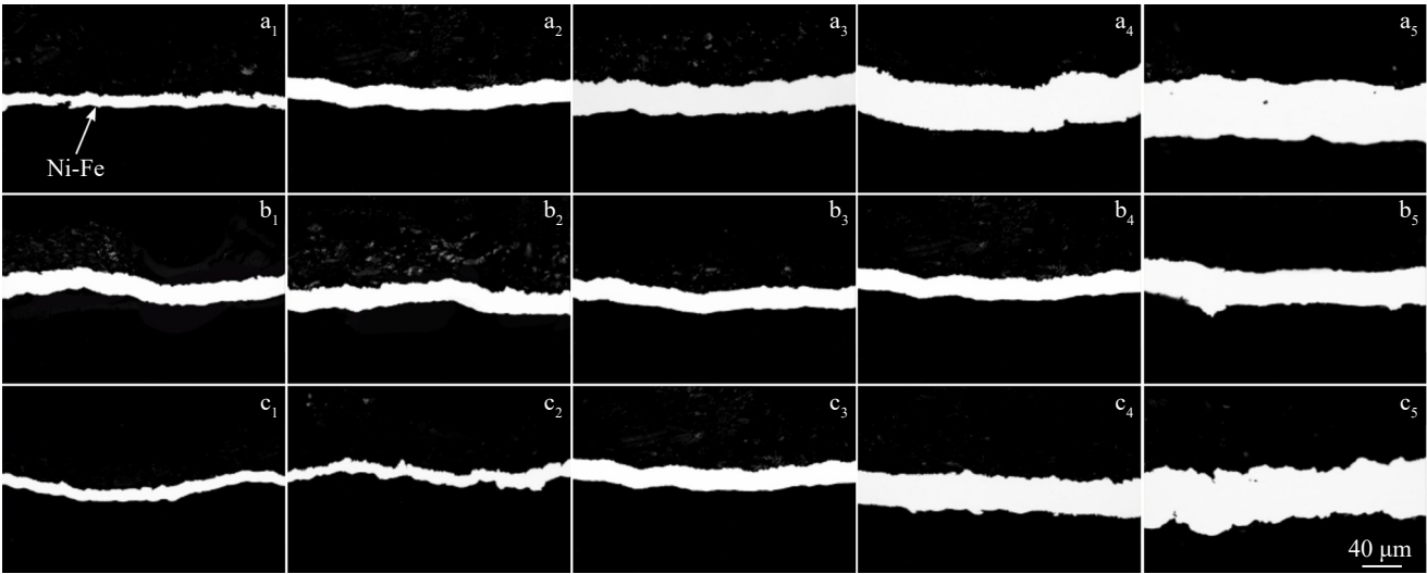
图 6 不同阴极电流密度、沉积温度和沉积时间下多孔 Ni-Fe 合金的沉积层截面形貌
