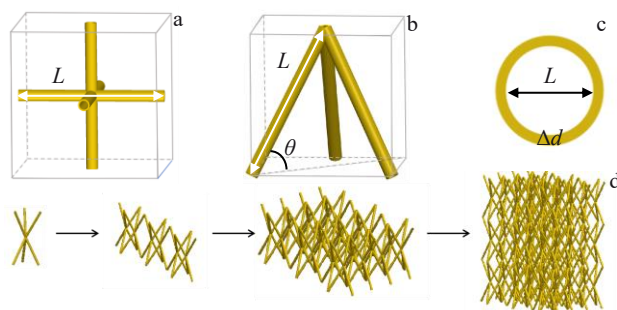
图 1 点阵结构建模示意图
